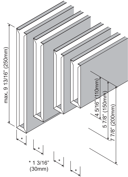
Fig. 145 Dimensions of the baffles
